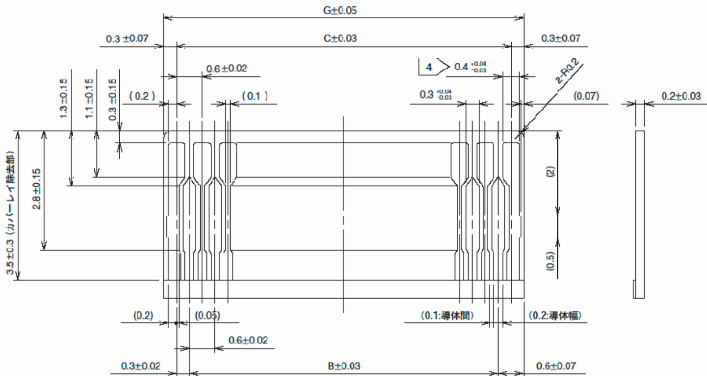
《寸法表》 単位：mm
