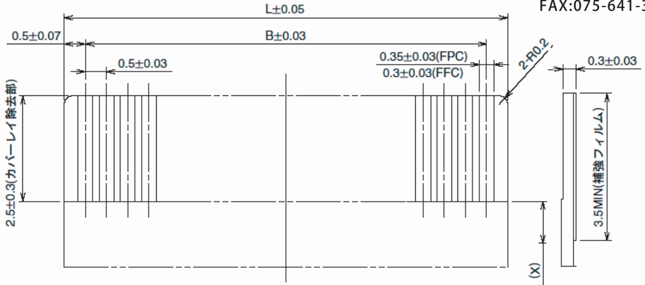
《寸法表》 単位：mm
